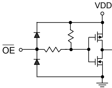
\overline{OE} Terminal
